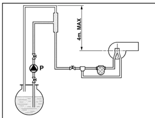
fig. 21 - Alimentazione ad anello
