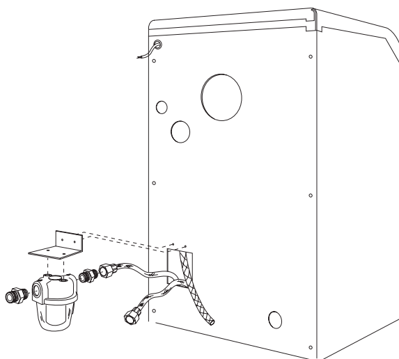
fig. 17 - Installazione filtro combustibile
