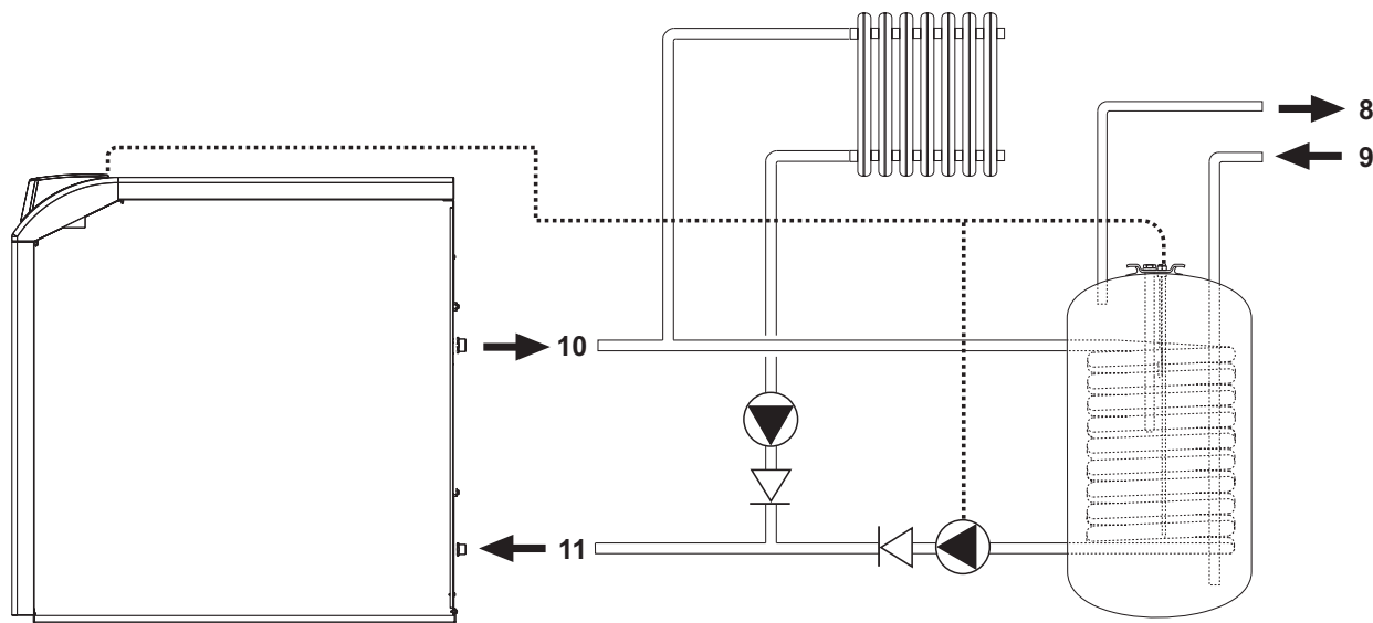
fig. 16 - Schema collegamento ad un bollitore esterno
