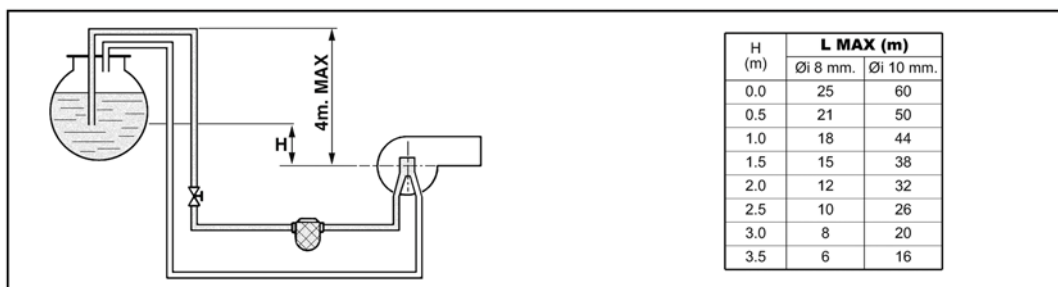
fig. 20 - Alimentazione a sifone
