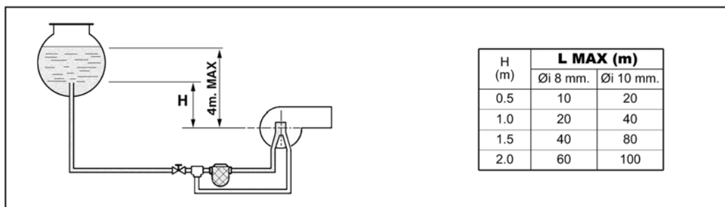
fig. 18 - Alimentazione per gravità
