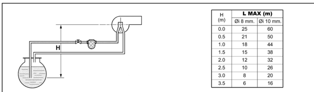
fig. 19 - Alimentazione per aspirazione
