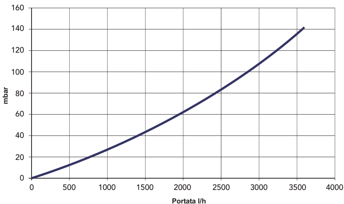
fig. 34 - Perdite di carico modelli 3 e 4 elementi
