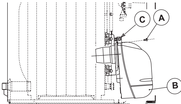
fig. 31 - Smontaggio bruciatore
