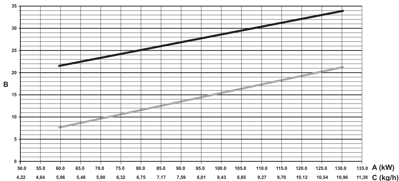
fig. 26 - Grafico regolazioni bruciatore SUN G10
