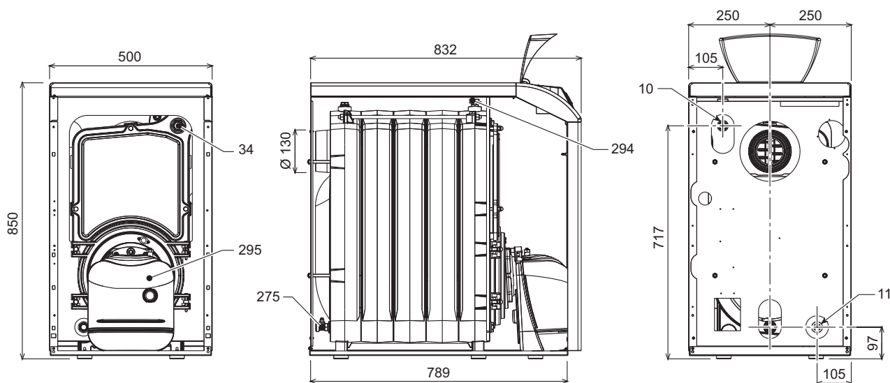
fig. 33 - Dimensionale attacchi e componenti principali versione 5 elementi
