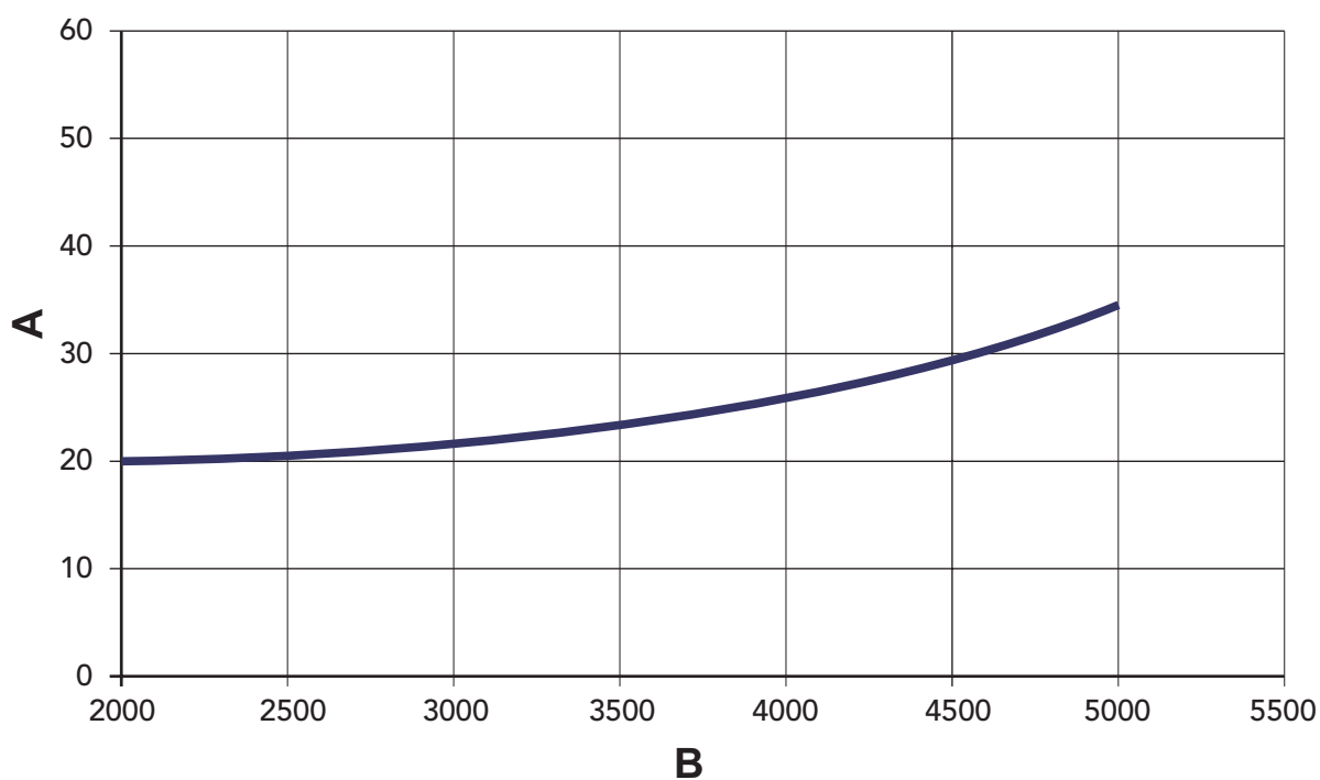
fig. 35 - Perdite di carico modelli 5 elementi
