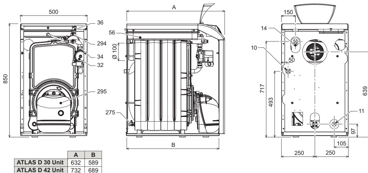
fig. 32 - Dimensionale attacchi e componenti principali versione 3 e 4 elementi
