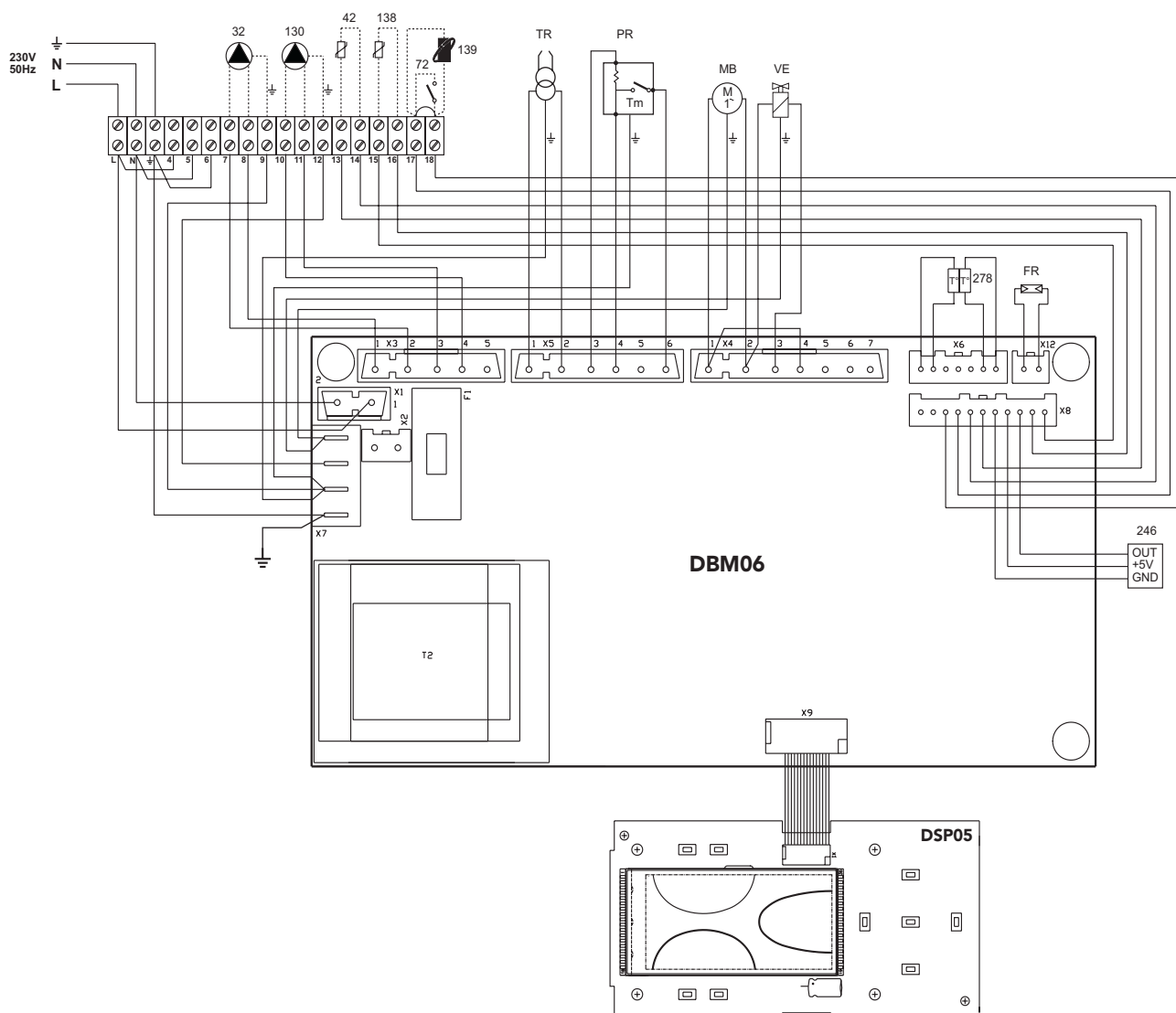
fig. 36 - Schema elettrico
